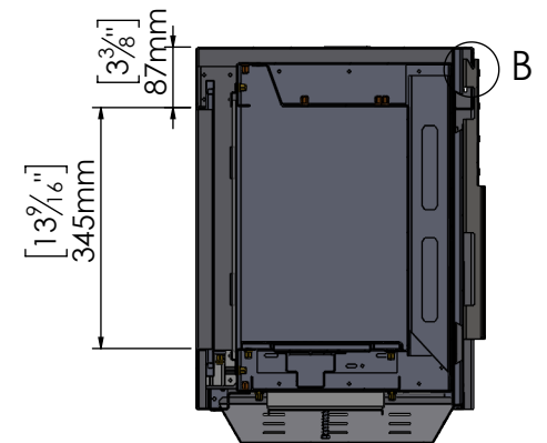
SECTION A-A SCALE 1 : 12
